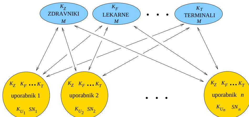
Slika 4: Delitev na skupine pri naši zdravstveni kartici. S K so označeni posamezni ključve, glavni ključ je označen z M . Vsak uporabnik ima tudi enolično serijsko številko SN_i .
