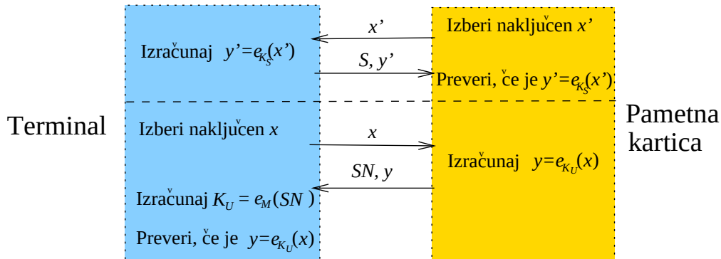
Slika 5: Pametna kartica predstavlja uporabnika, terminal pa skupino. Z e_K označimo šifrirno funkcijo s ključem K . Le-ta pretvori s pomočjo ključa K vsebino v oklepaju v šifrirano besedilo. V zgornjem delu terminal overi pametno kartico s pomočjo glavnega ključa M in serijske številke kartice ( SN ), v spodnjem delu pa kartica overi terminal s pomočjo skupinskega ključa K_S . Kartica vsebuje samo K_U in K_S ne pa tudi M , medtem ko terminal ne pozna K_U , ampak ga izračuna s pomočjo M .
